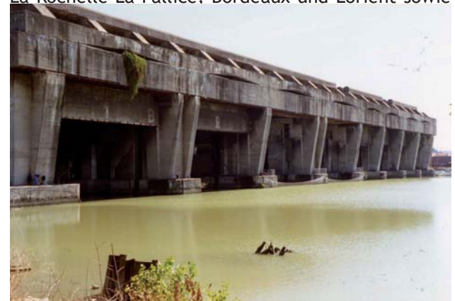
U-Bootbunkeranlage in Brest
