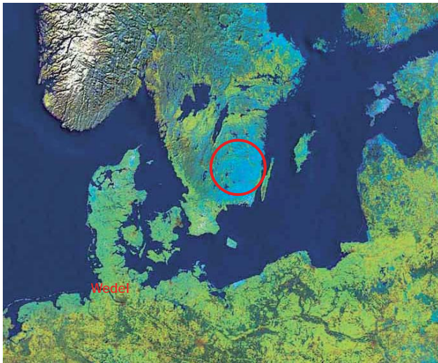
Herkunftsgebiet der Småland-Granite
